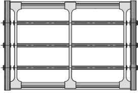
Yatay Separatör Uygulaması Horizontal Separator Application
